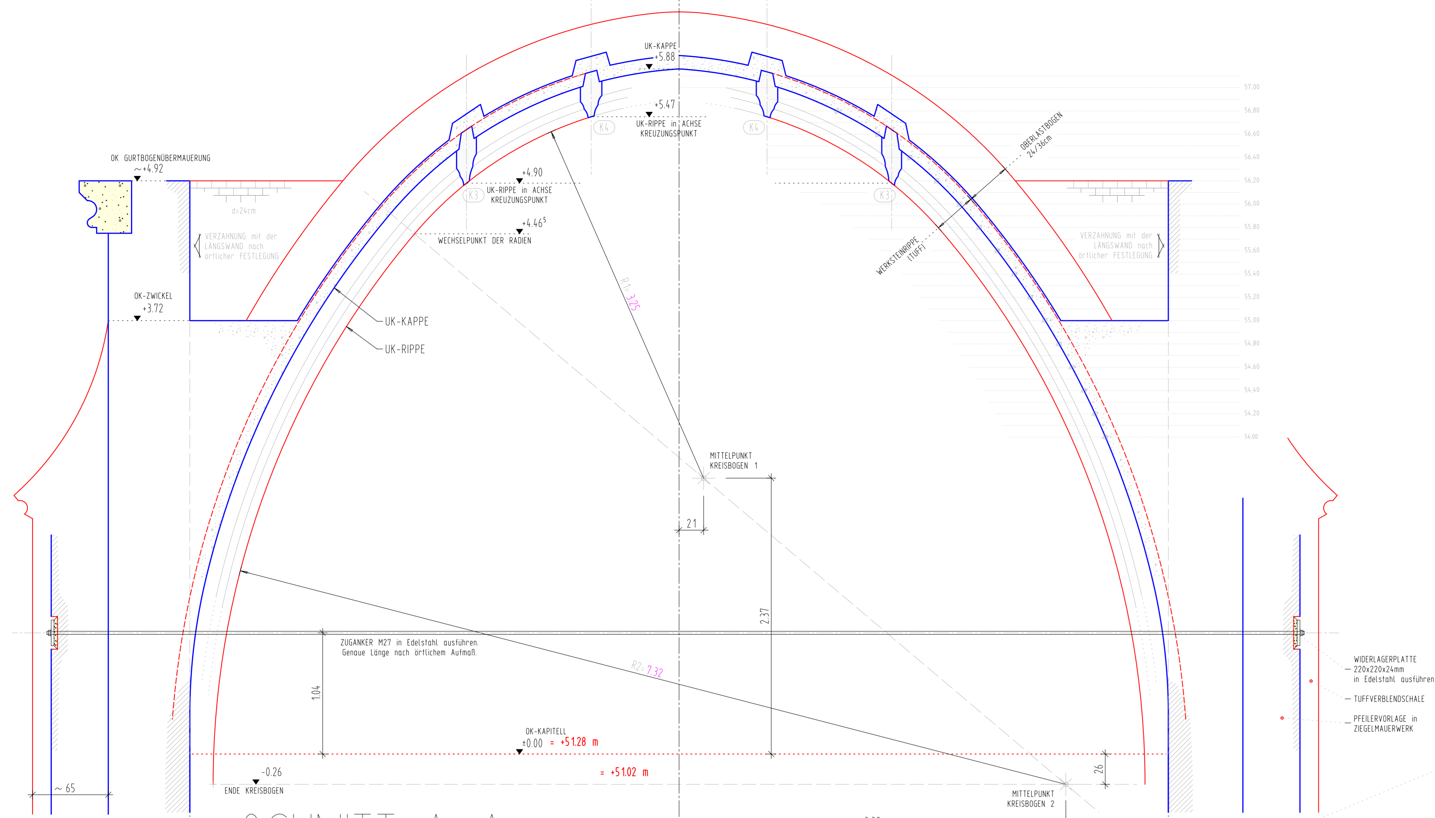
SCHNITT A-A GURTBOGEN
